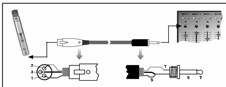
Fig. 3: Conexão através de um cabo desbalanceado
