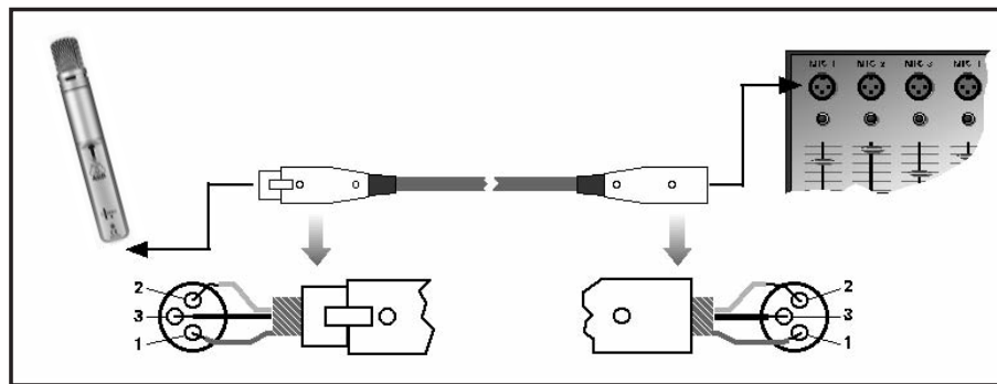
Abb. 2: Anschluss über symmetrisches XLR-Kabel
