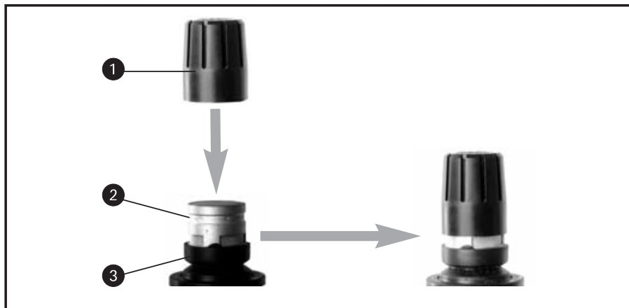
Fig. 5 : Montage du PPC 1000/PB 1000.
