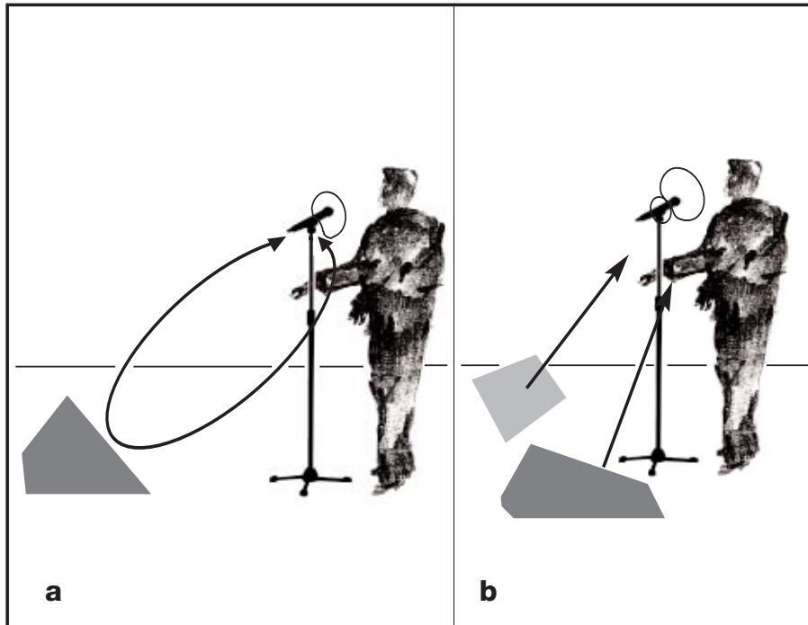
Abb. 7: Mikrofon-aufstellung für minimale Rückkopplung
