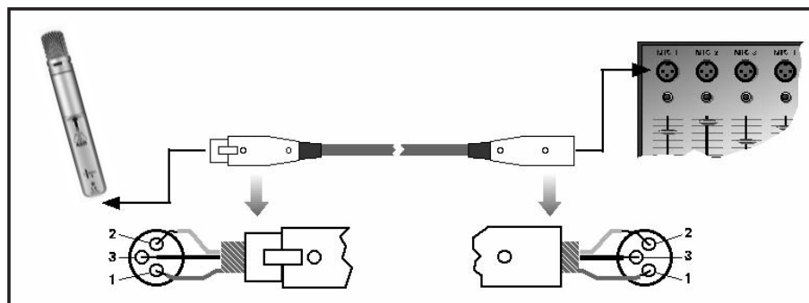
Abb. 4: Anschluss an symmetrischen Eingang mit Phantomspeisung
