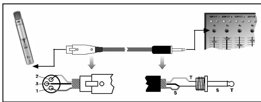
Fig. 3: Collegamento tramite cavo asimmetrico
