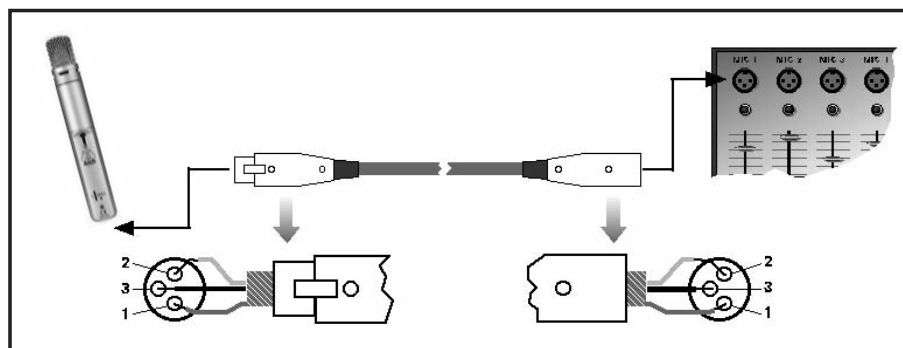
Fig. 2: Collegamento tramite cavo XLR simmetrico
