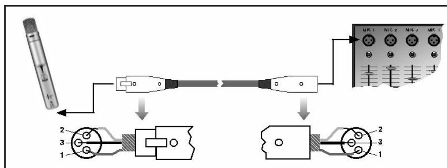
Fig. 4 : Branchement sur entrée symétrique avec alimentation fantôme.
