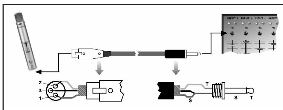
Fig. 3: Conexión con cable no balanceado
