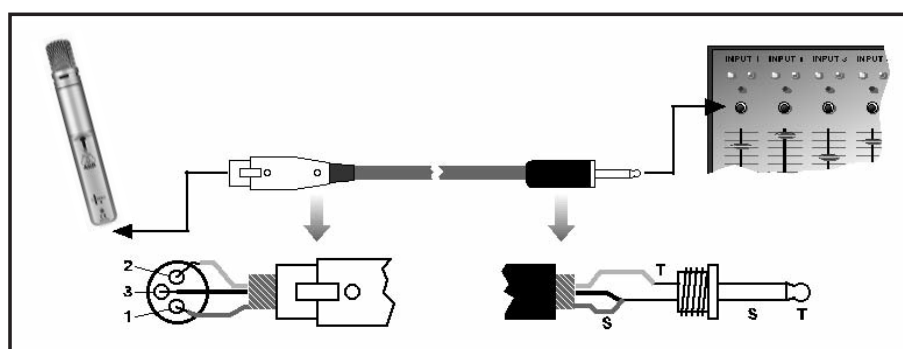
Fig. 3 : Raccord à l'aide d'un câble asymétrique
