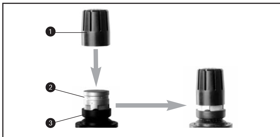
Fig. 5: Montagem do PPC 1000/PB 1000
