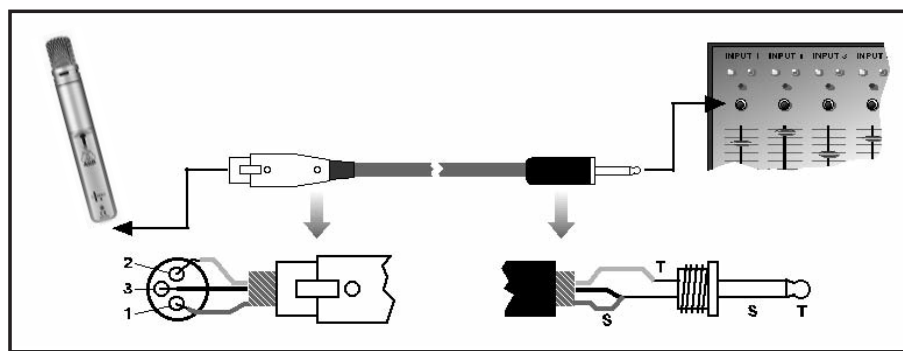
Abb. 3: Anschluss über unsymmetrisches Kabel
