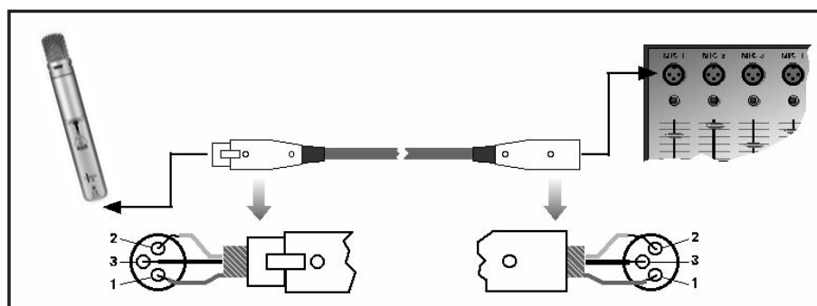
Fig. 4: Conexão a uma entrada balanceada com alimentação fantasma
