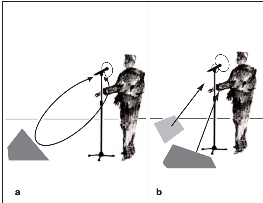
Fig. 7: Emplazamiento del micrófono para prevenir la retroalimentación
