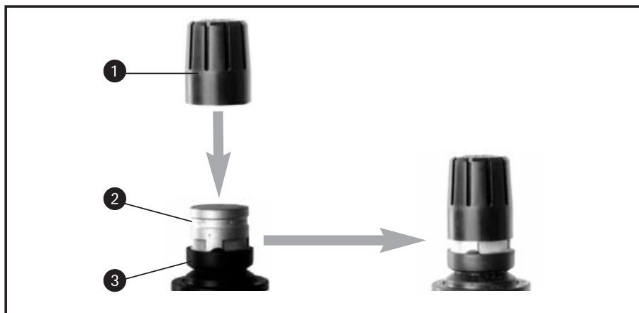
Abb. 5: PPC 1000/ PB 1000 montieren.
