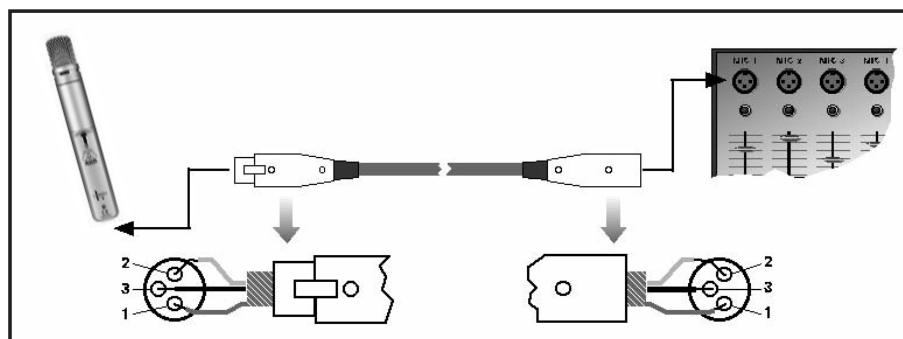
Fig. 4: Collegamento ad uscita simmetrica con alimentazione phantom
