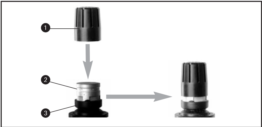
Fig. 5: Come montare il PPC 1000/PB 1000.
