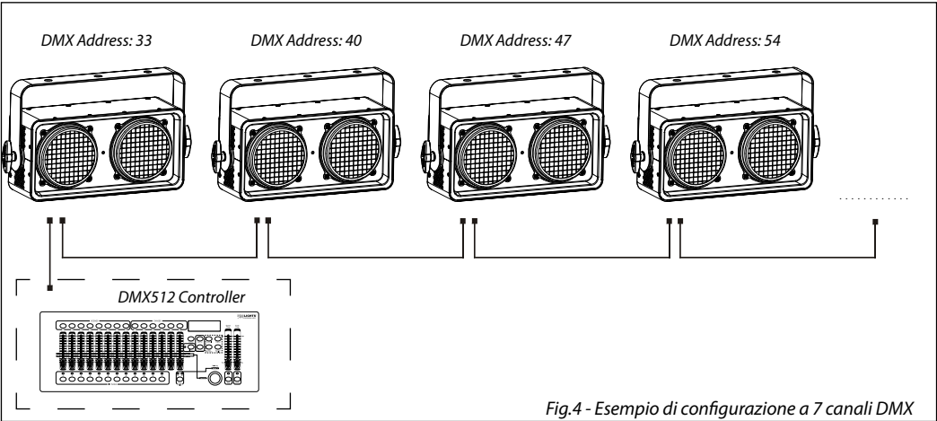
Fig.4 - Esempio di configurazione a 7 canali DMX
